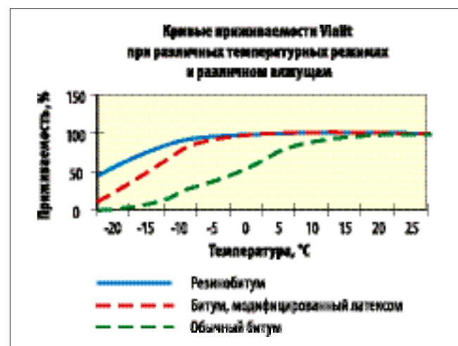
Рис. 15. Приживаемость щебня в резинобитумном вяжущем.
