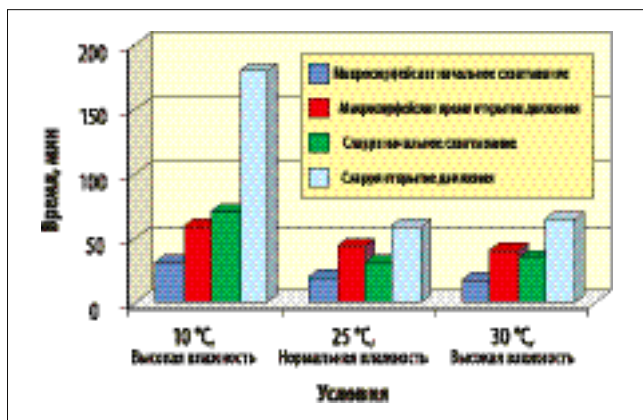
Рис. 5. Влияние времени, температуры и влажности на скорость набора прочности покрытий Сларри Сил и Микросюрфейсинг.
