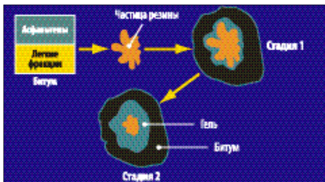
Рис. 8. Стадии реакции частиц резины и битума.
