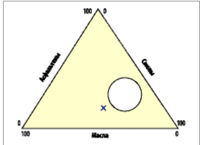
Рис. 3. Оценка химического состава битума.
