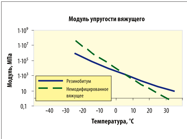
Рис. 10. Улучшение термической чувствительности при добавлении резины.
