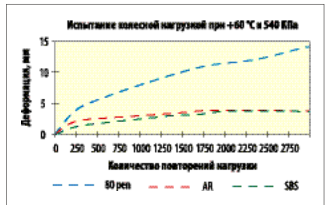
Рис. 18. Устойчивость смесей на основе резинобитума к деформациям..
