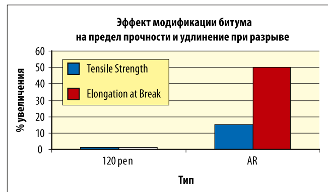
Рис. 14. Влияние модификации битума на предел прочности на разрыв и удлинение при разрыве – тест Бенсона.
