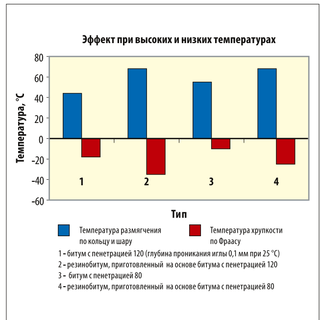
Рис. 11. Влияние на температуру размягчения по кольцу и шару и температуру хрупкости по Фраасу.
