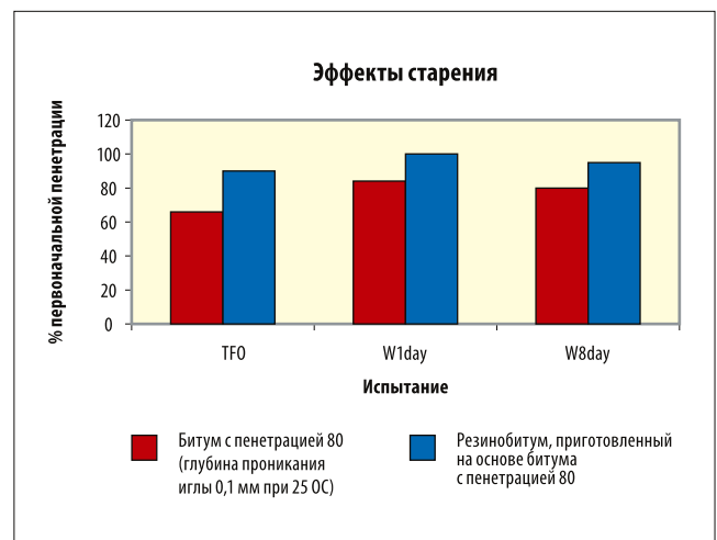
Рис. 12. Эффекты старения резинобитумных вяжущих (в печи – TFO, в симуляторе погодных условий – W).
